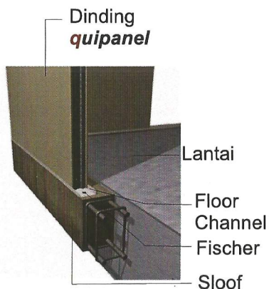
Detail sambungan panel dengan Sloof
