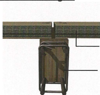
Sambungan lantai quipanel dengan balok beton
