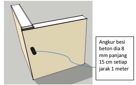
Gambar 1. Sambungan sudut
