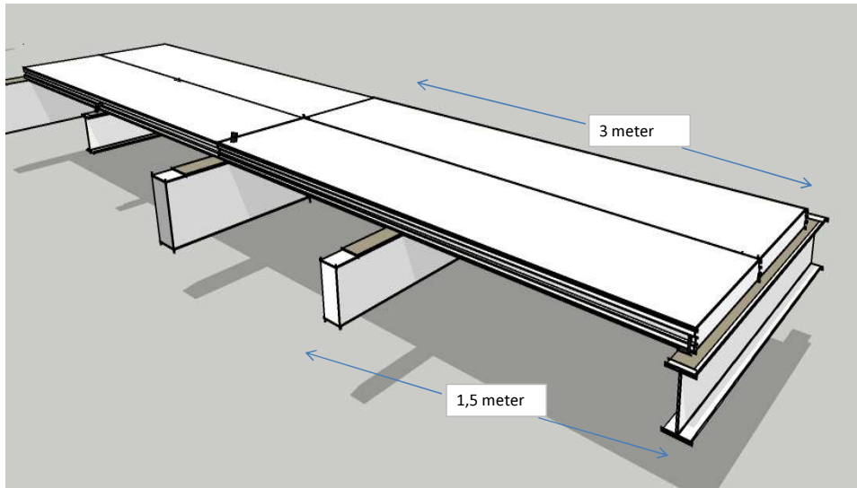
Cara pemasangan lantai quipanel
