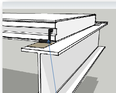
Cara pemasangan lantai quipanel
