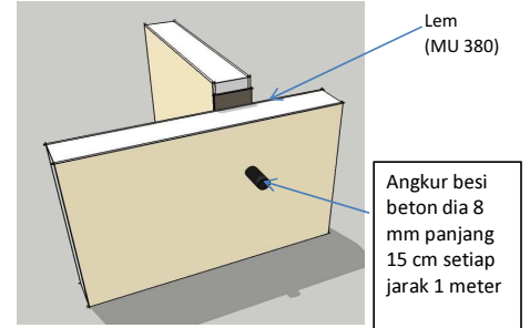
Gambar 2. Sambungan T
