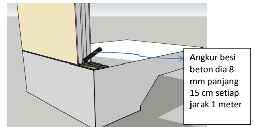
Gambar 4. Sambungan panel dan sloof
